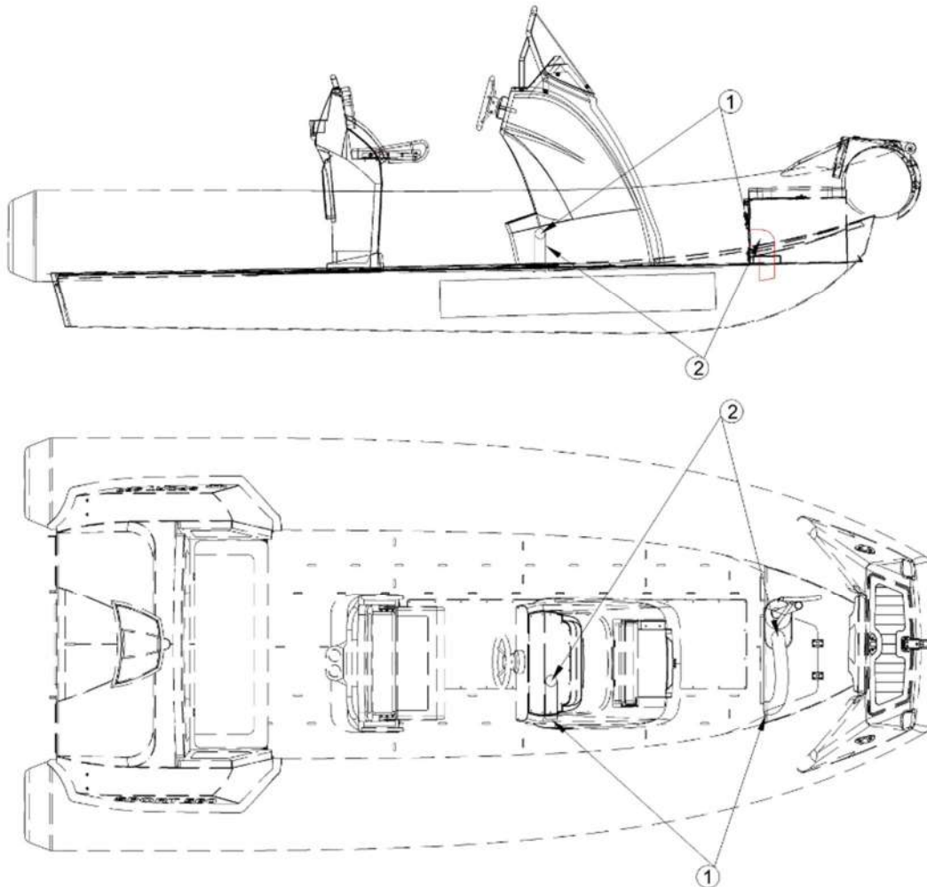
Darstellung der Tankraumbelüftung
